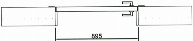
顶视图
