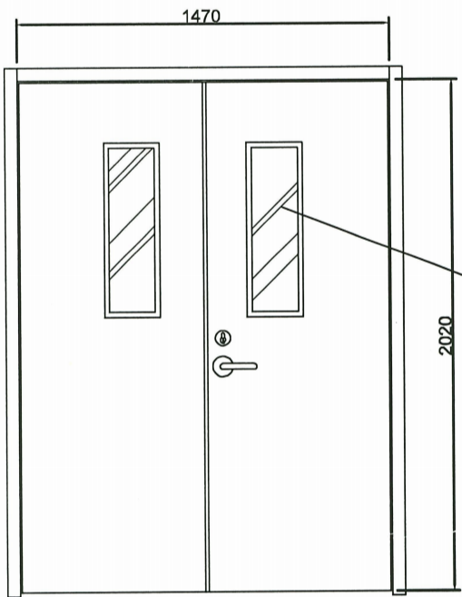
正面图
