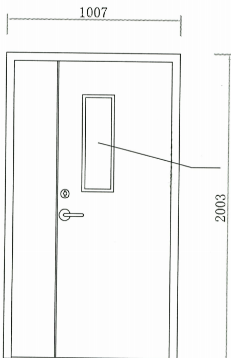
正面图
