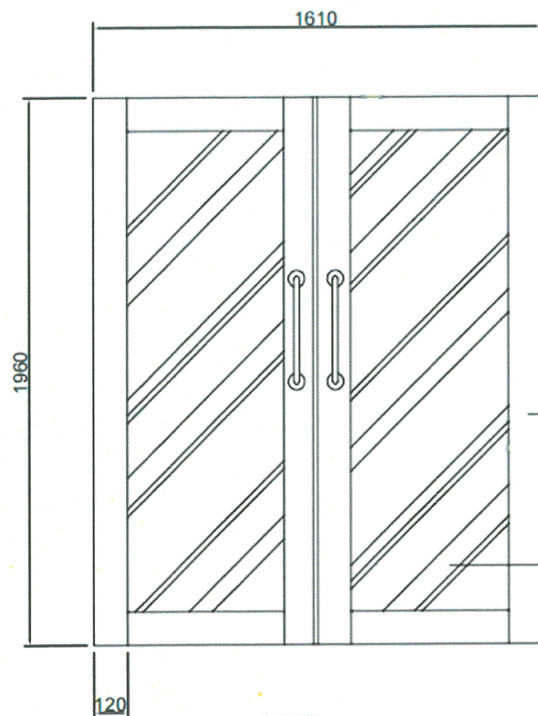
正面图
