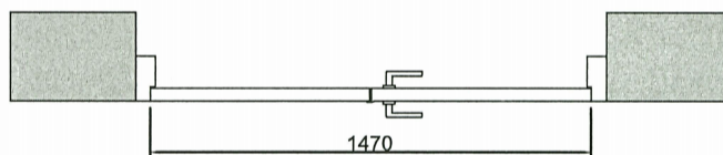
顶视图
