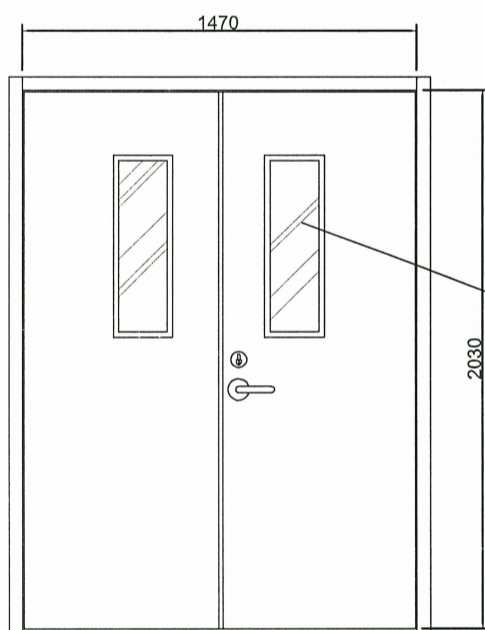
正面图
