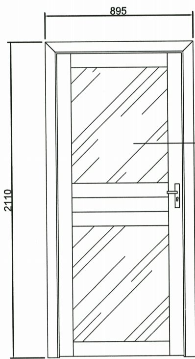
正面图
